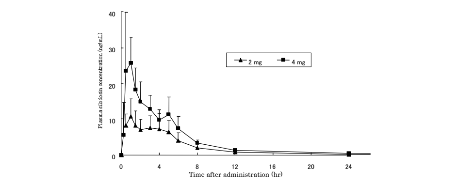
圖1. 健康成年男子於空腹分別投與2 mg與4 mg後，Silodosin 的血中濃度變化情況，數據以平均值±標準差表示(6例)。
